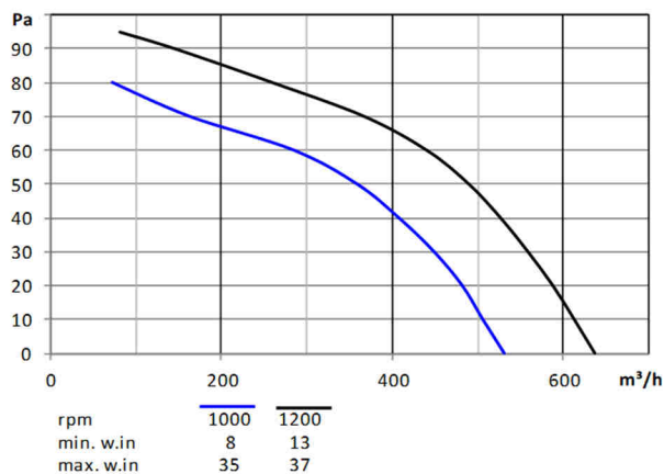
FAS145P.15EB.. 1200 / 1000rpm
