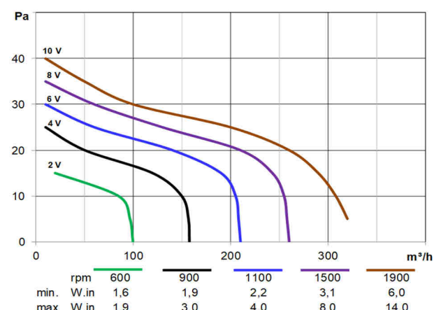
ETD60300EC15 1900÷600rpm
