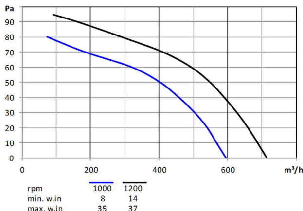
FAS145P.15EB.. 1200 / 1000rpm
