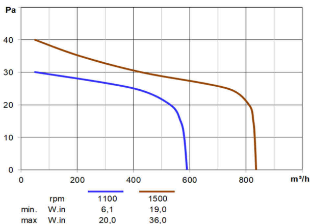
ETD60605EB21 1500/1100rpm
