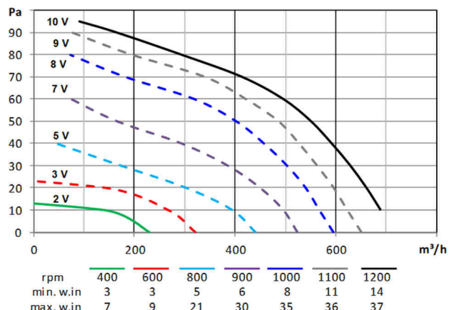
FAS145P.15EC.. 1200 ÷ 400rpm
