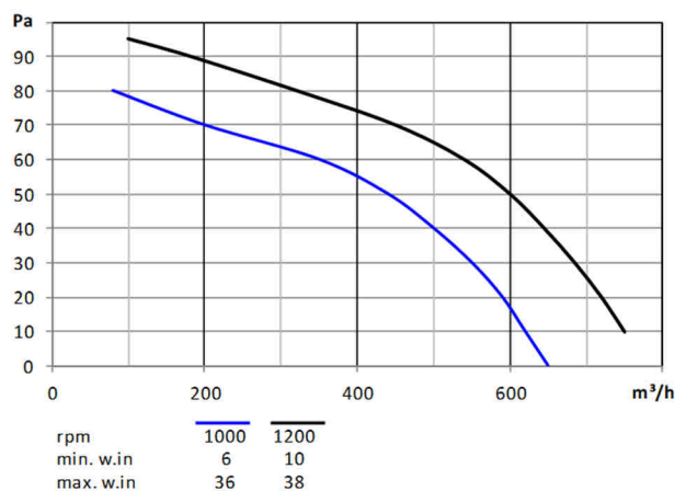
FAS145Q.15EB.. 1200 / 1000rpm
