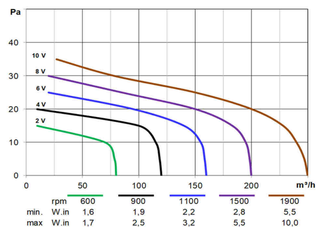
ETD60240EC15 1900÷600rpm
