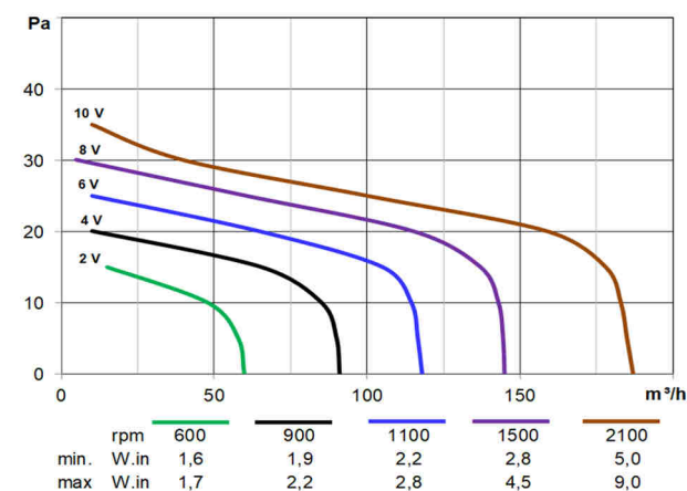
ETD60180EC15 2100÷600rpm
