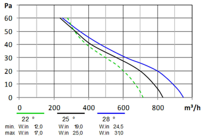
15UA ... Ø254
