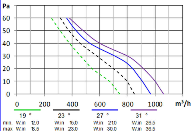
21UA ... Ø254
