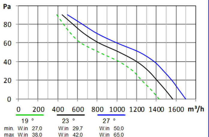
21UA ... Ø300
