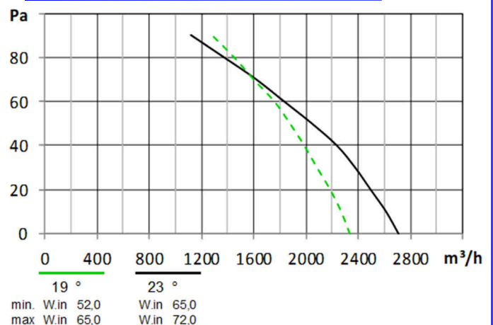
21UA ... Ø350
