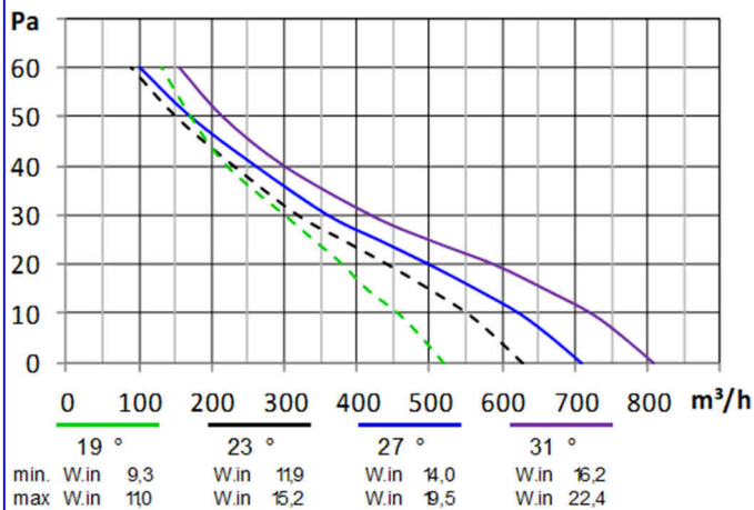
21UA ... Ø230
