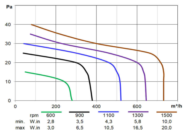
ETD80505EC15 1500÷600rpm
