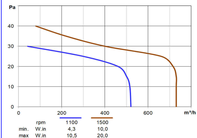
ETD80505EB15 1500/1100rpm
