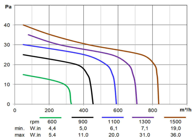
ETD60605EC21 1500÷600rpm
