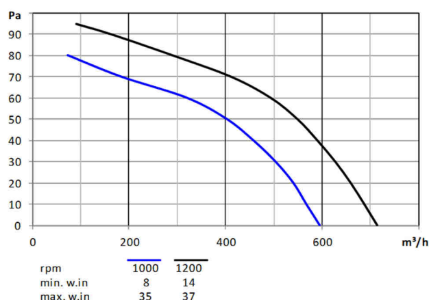
FAS145P.15EB.. 1200 / 1000rpm
