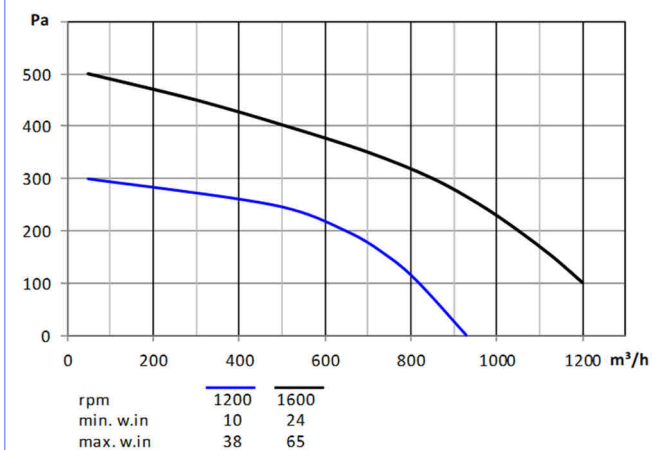
FAS145Q.21EB.. 1600 / 1200rpm
