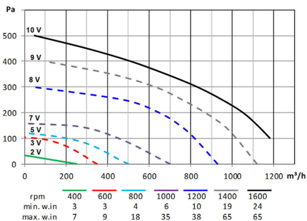
FAS145Q.21EC.. 1600 ÷ 400rpm
