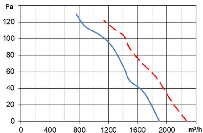
ER4L331U. ø 315/31° — 50Hz — 60Hz
