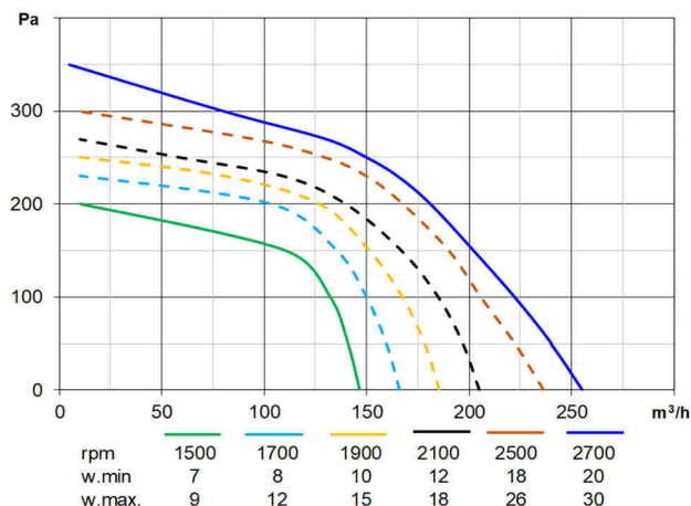
OSX(D)120B.15EC.. 2700÷1500rpm
