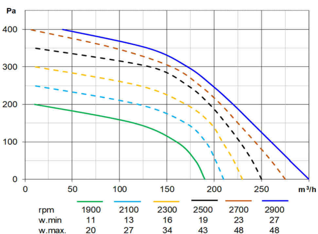
OSX(D)133B.21EC.. 2900÷1900rpm
