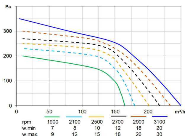
OSX(D)108B.15EC.. 3100÷1900rpm
