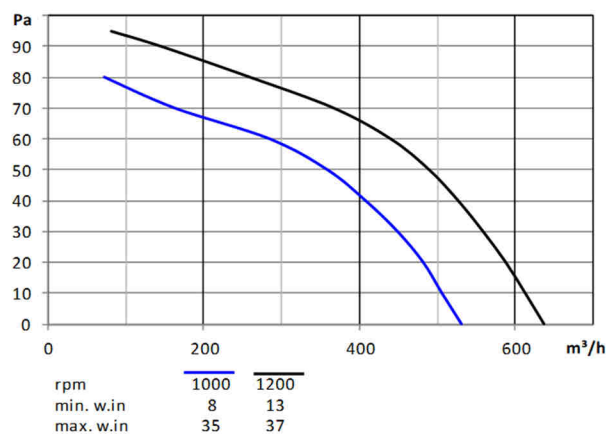
FAS145P.15EB.. 1200 / 1000rpm
