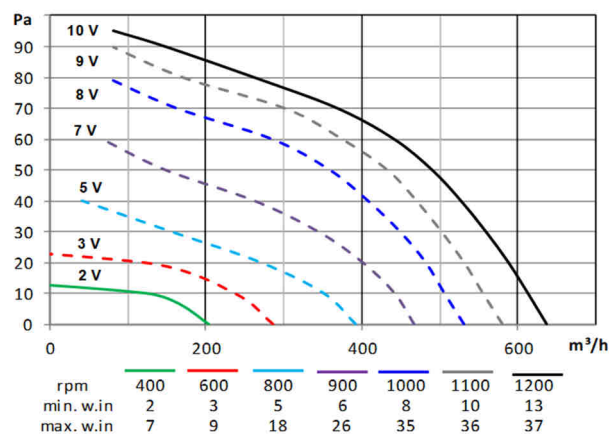
FAS145P.15EC.. 1200 ÷ 400rpm
